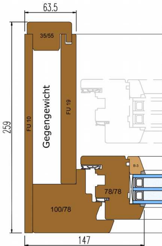
Schnitt A-A
