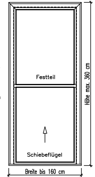
OpenAir-SV-Dachschiebefenster -zweiteilig- ein Schiebeflügel
