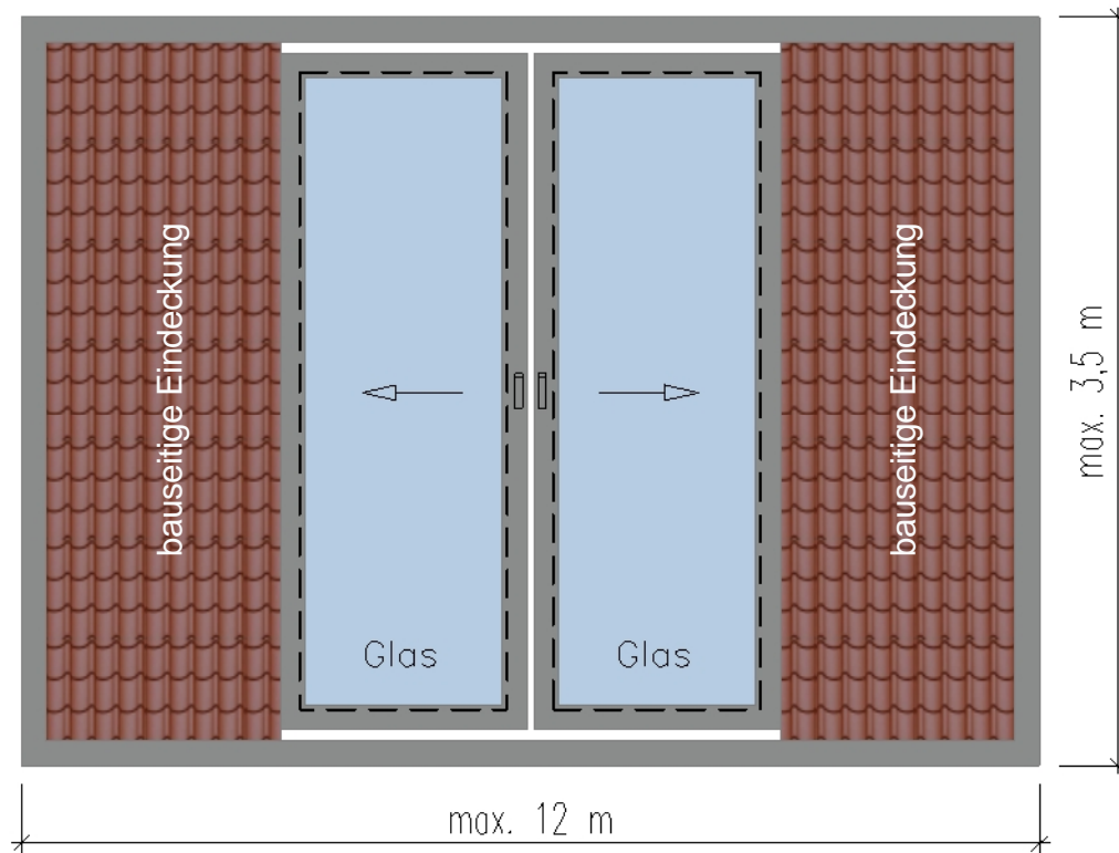
Panorama-Dachschiebefenster (Typ AH 4-teilig) -Doppelflügel (Stulpanlage)-
