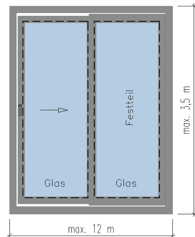
Panorama-Dachschiebefenster (Typ AL 2-teilig)
