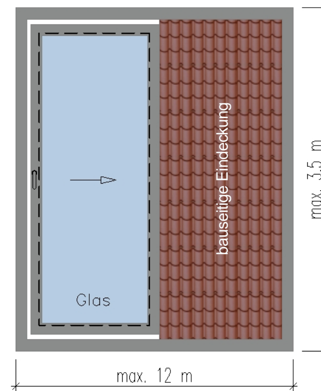
Panorama-Dachschiebefenster (Typ AH 2-teilig)
