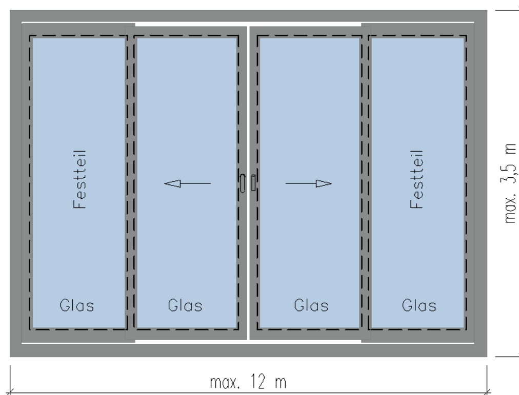
Panorama-Dachschiebefenster (Typ AL 4-teilig) -Doppelflügel (Stulpanlage)-
